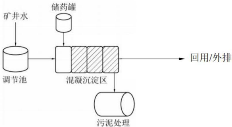
图 4-1 混凝处理原理示意图
