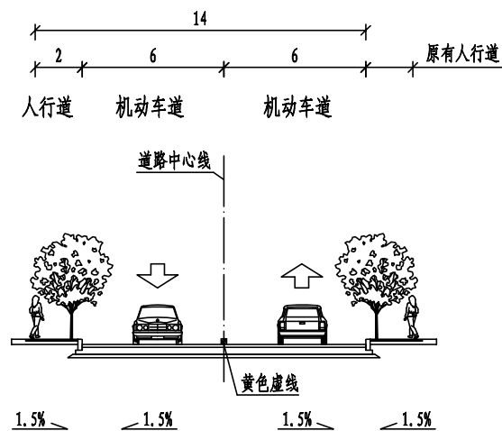
标准横断面图
