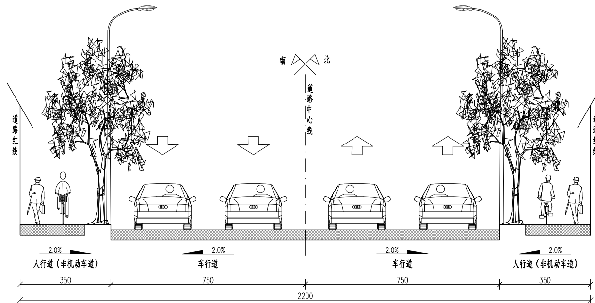
道路标准横断面图 红豆杉路（推荐断面）
