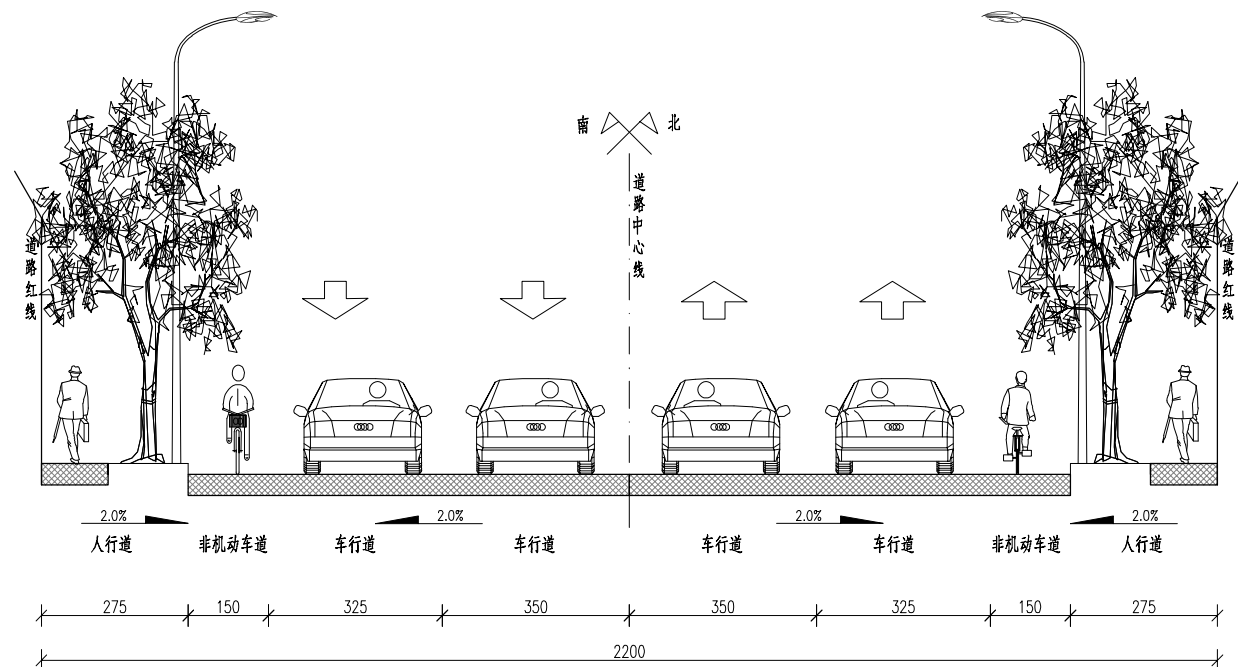
道路标准横断面图 红豆杉路（比选断面）
