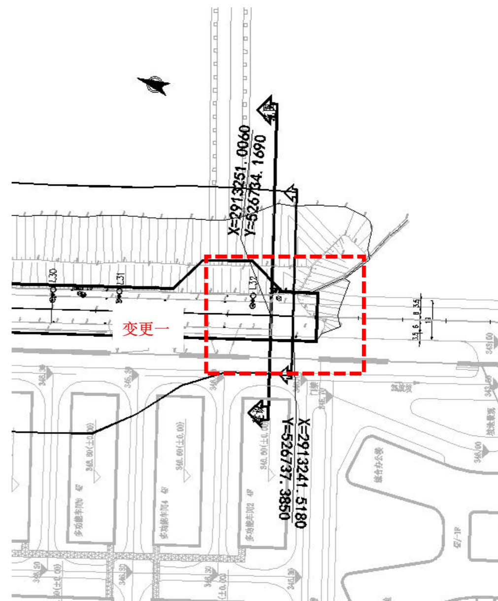
变更一：路面实施至 K1+420 末端预留 10m 路面，便于后期衔接实施
