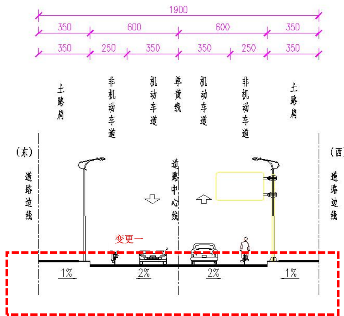
交通安全设施标准横断面图
