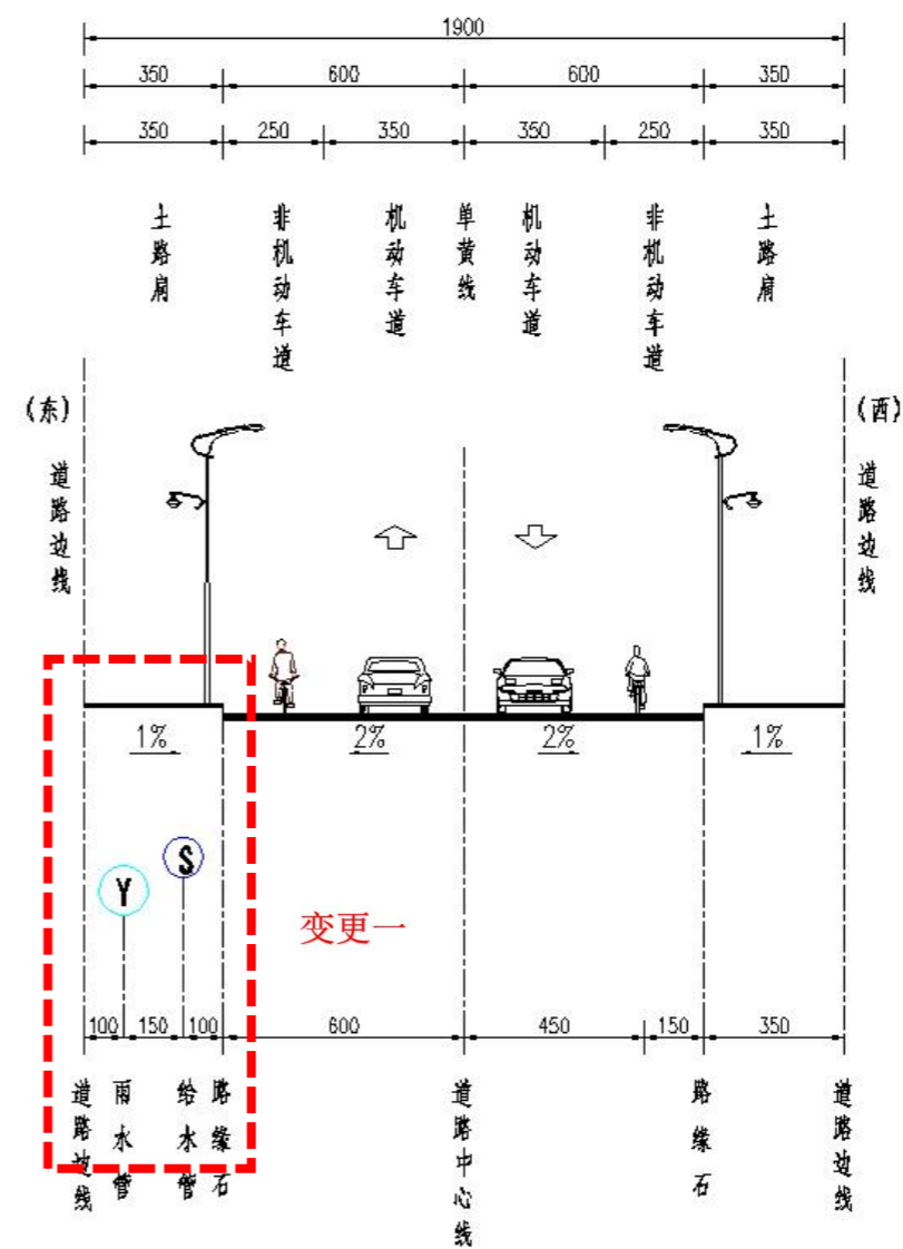
管综标准横断面图
