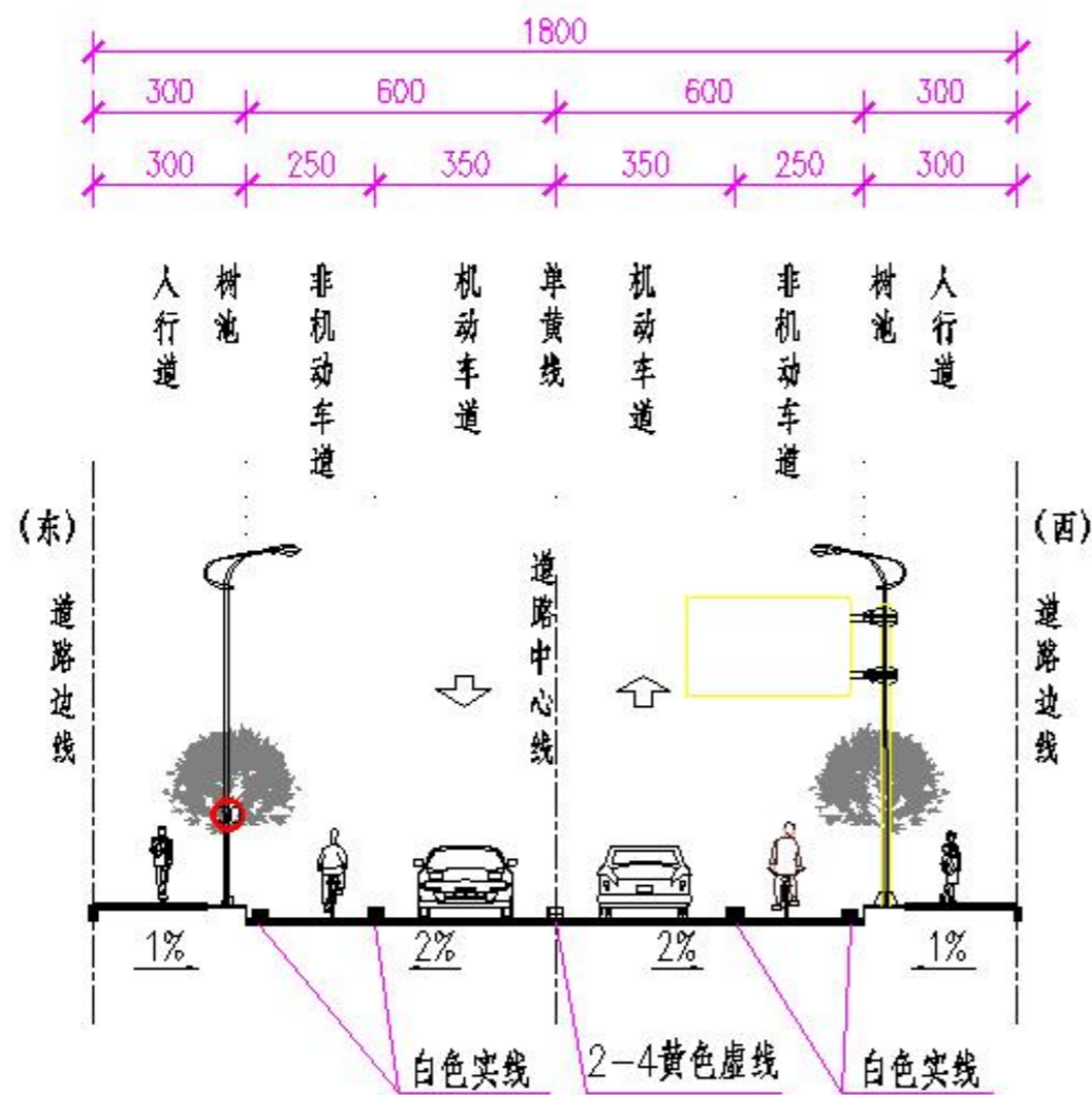
交通安全设施标准横断面图
