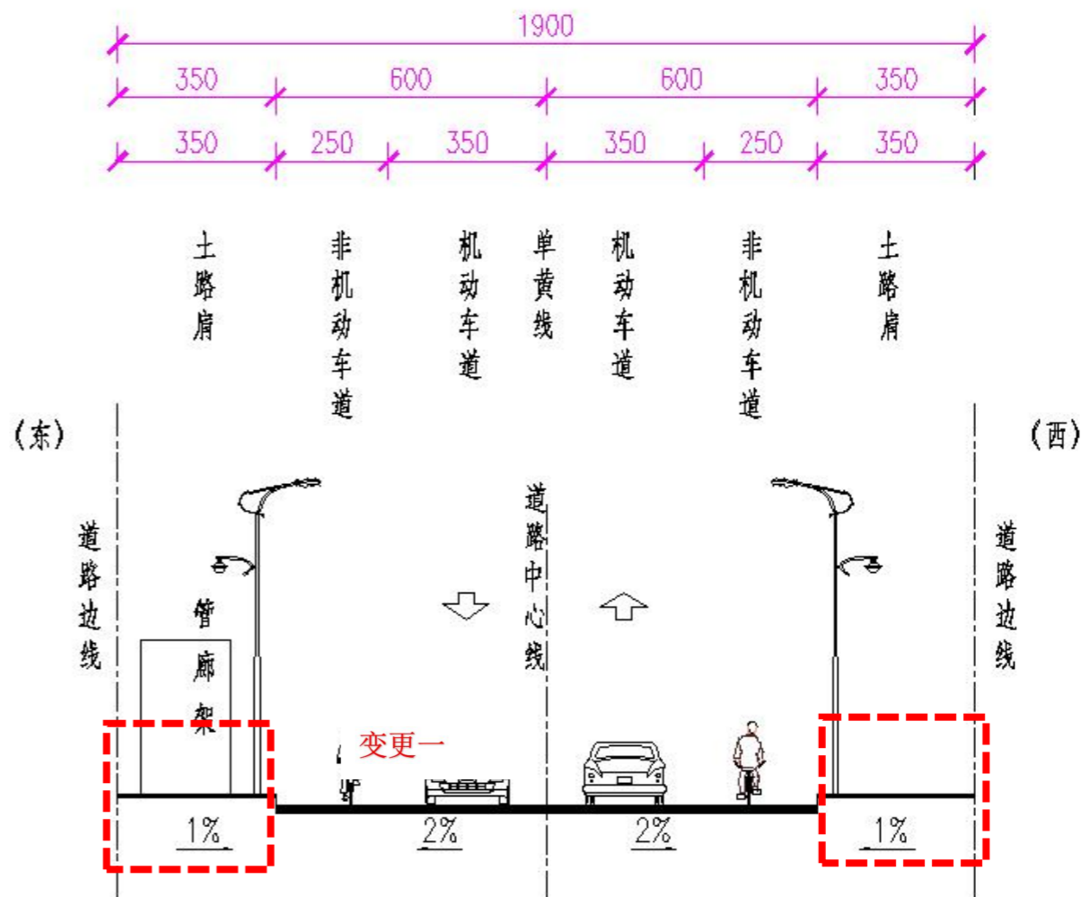
道路标准横断面图
