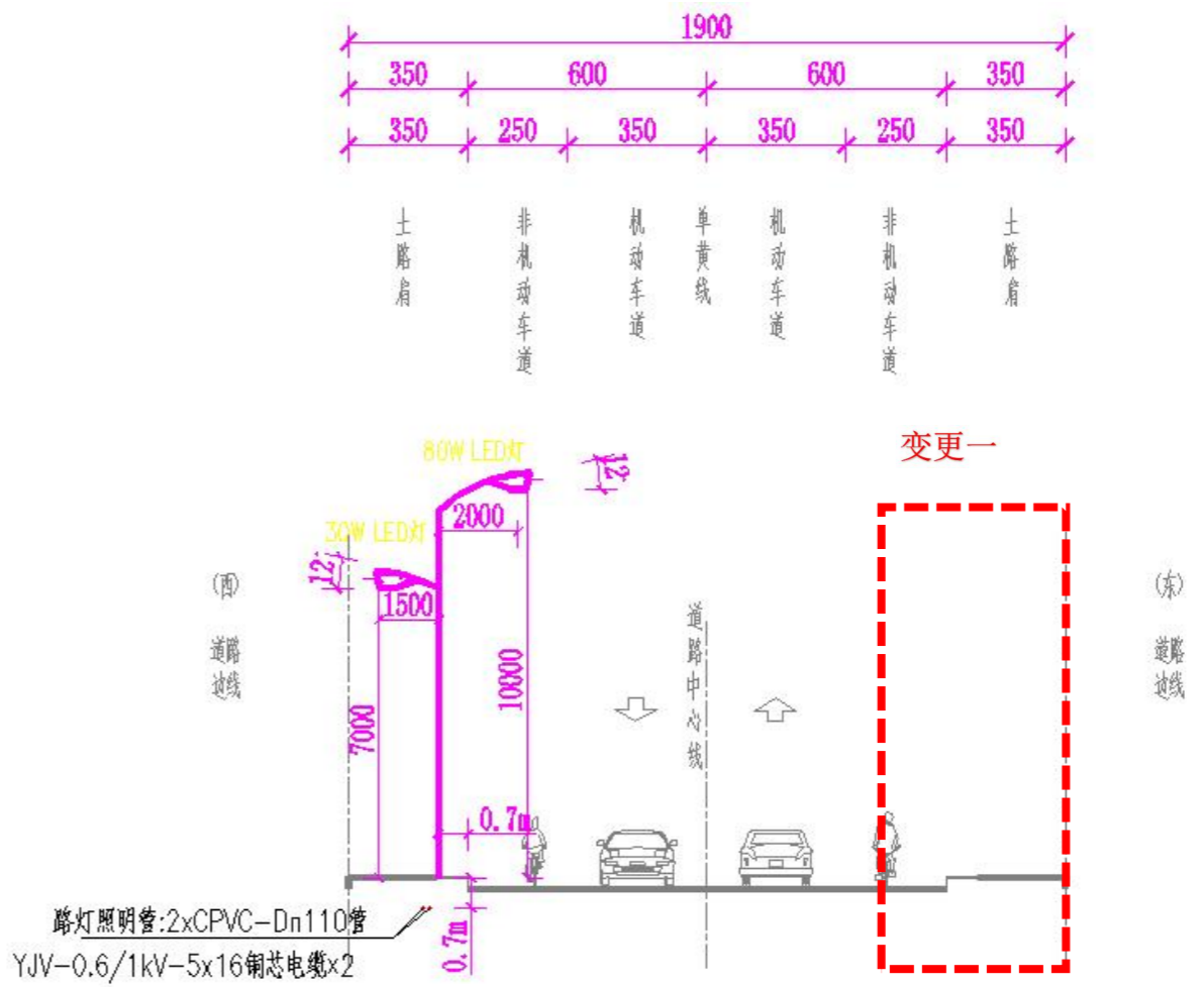
路灯布置横断面设计图
