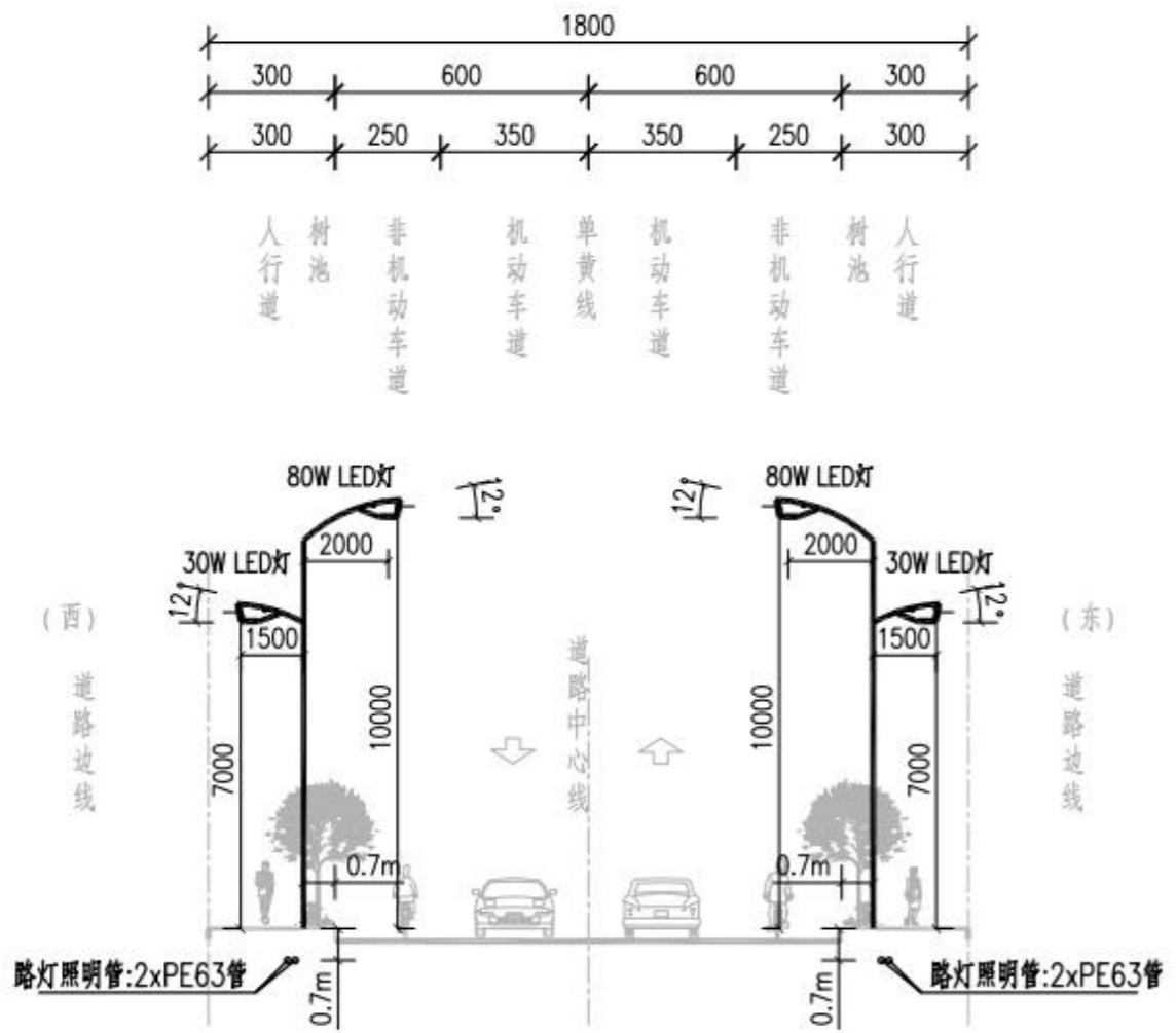
路灯布置横断面设计图 (K0+300~K1+430)
