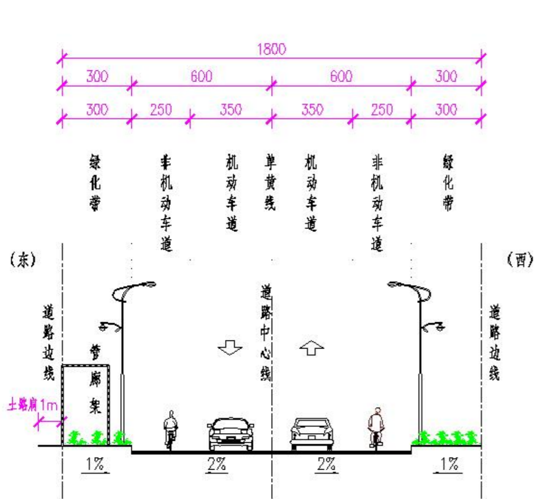
道路标准横断面图
