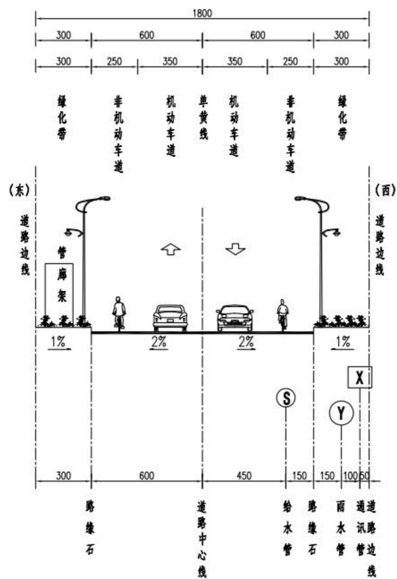
管综标准横断面图
